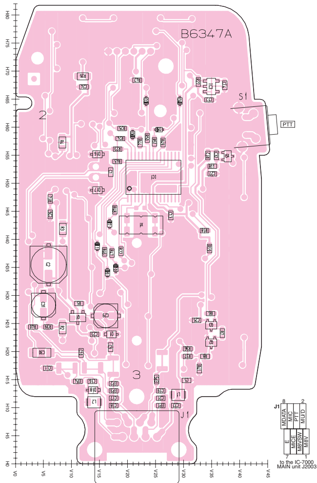
• BOTTOM VIEW (HM-151)
